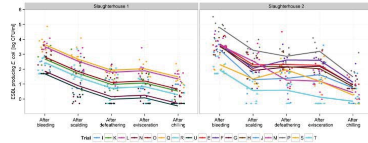
Figuur 5.11.1. Dynamiek in ESBL-concentraties op karkassen van vleeskuikens tijdens het slachtproces in twee slachthuizen (naar Pacholewicz E, et al. 2015).
