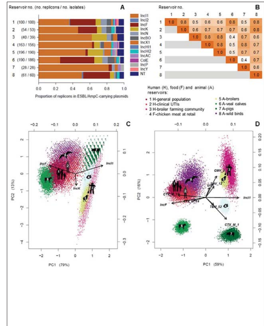
Figuur 4.1.2. A: Relatieve verdeling van plasmid varianten aangetoond in 8 reservoirs. B: Proportionele similariteit in plasmiden tussen de 8 reservoirs (0 is geen overeenkomst en 1 is identiek). C: Principale Componenten Analyse op basis van bootstrap waarbij de overeenkomsten en verschillen in de verdelingen worden gevisualiseerd. D: PCA van ESBL-Plasmid combinaties per reservoir (met toestemming uit Dorado Garcia et al, 2017).
