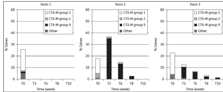
Figuur 5.6.1. Dynamiek in ESBLs in drie vleeskalverbedrijven (Hordijk, Mevius et al, 2013)
