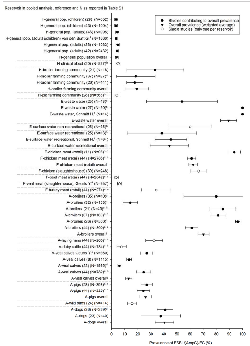
Figuur 4.1. Prevalentie (%) van genetisch bevestigde ESBL/(AmpC) producerende E. coli per bron (met toestemming uit Dorado-García et al. 2017; voor referenties zie Tabel Supplement 1).
