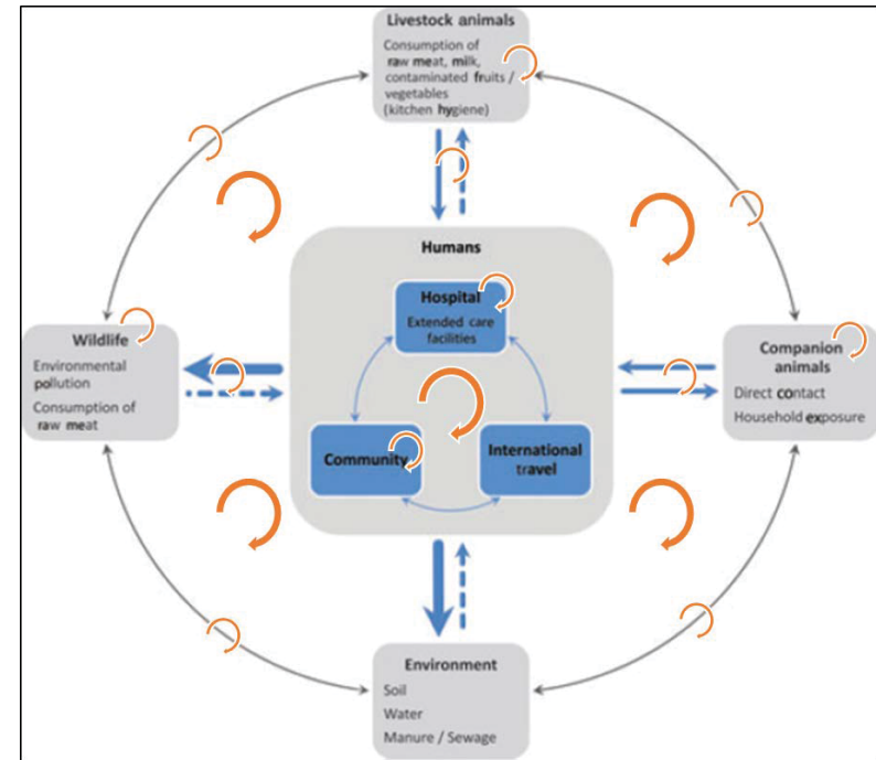
Figuur 4.3.1. De dynamiek van de transmissie van ESBLs tussen verschillende reservoirs (naar Ewers et al, 2012)
